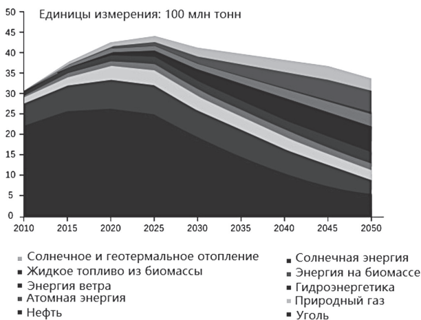
Рис. 3. Потребление энергии в Китае (2010–2050 гг.) 8
